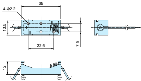
N cell×1
