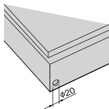
〔取付穴寸法〕
