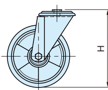
CAF5-FSL
