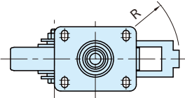
CAF5-PSL
