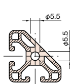
断面 A-A (2ヶ所)
