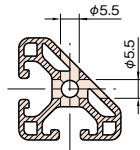
断面 A-A
