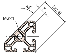
断面 B-B (2ヶ所)
