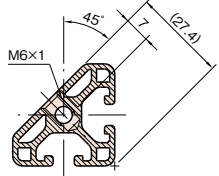
断面 B-B (2ヶ所)
