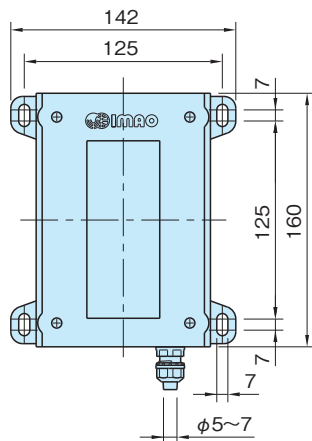
FW-SST02 (送信機)
