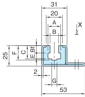
CGOC-A (Aタイプ)
