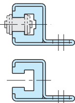
CGOC60Bの溝形状
