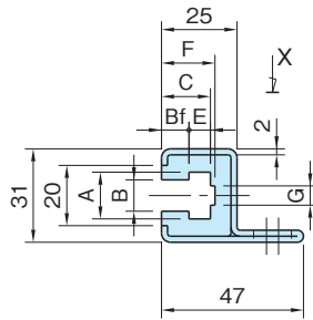
CGOC-B (Bタイプ)
