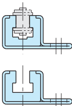
CGOC60Aの溝形状
