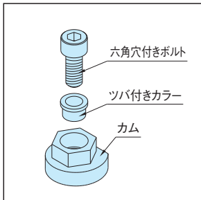
部品構成
