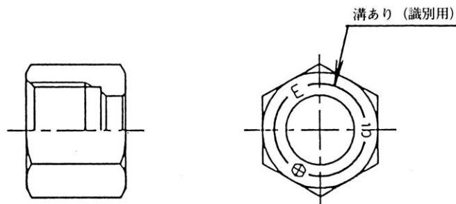
エンベロープ付スリーブ用ナットの識別表示
