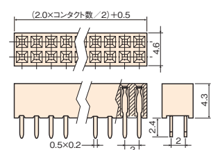
ソケット(HTW-20043-00S)
