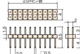
ピン(HTW-20058-00P)
