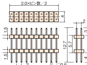
ピン(HTW-2010-00P)
