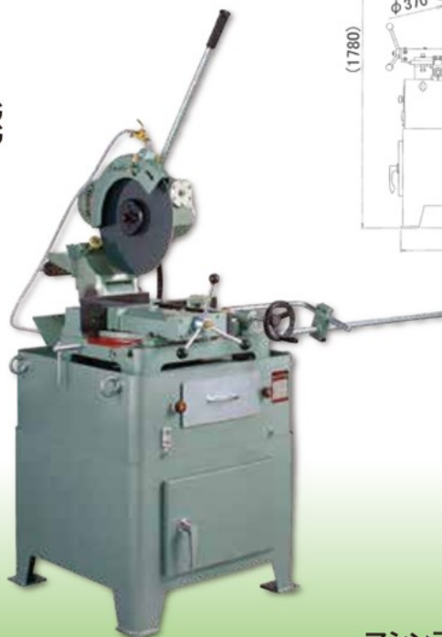
マシンテーブル取付例
